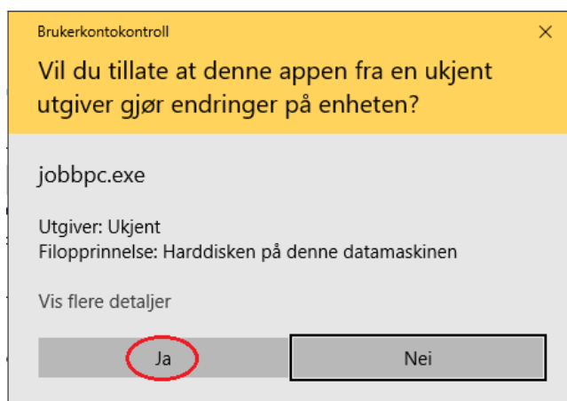
Figur 1 - Brukerkontroll
